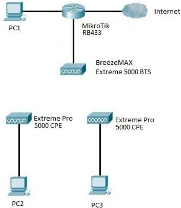
Figura 4.2 Topología utilizada para las pruebas
