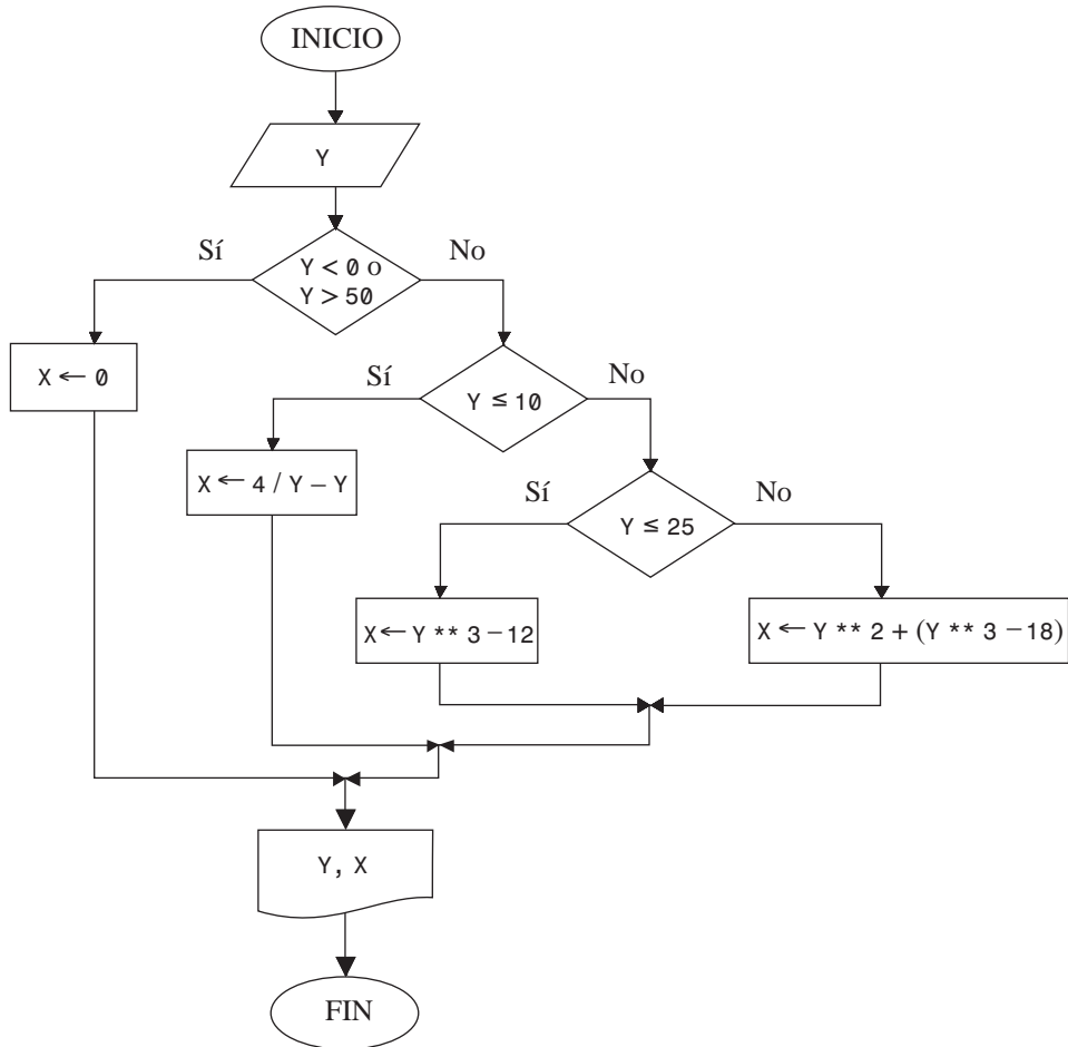
Diagrama de flujo 2.13
